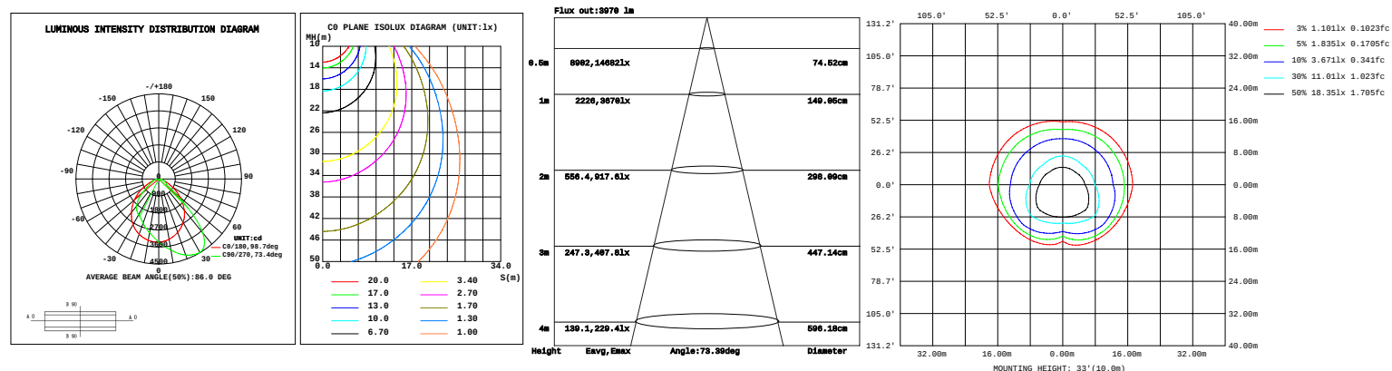
CIP-FWP2842567W27-345K (56W & 40000K)
