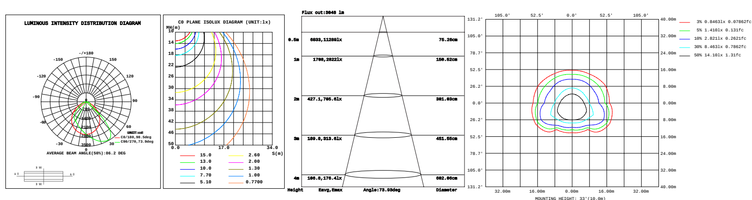
CIP-FWP2842567W27-345K (42W & 40000K)
