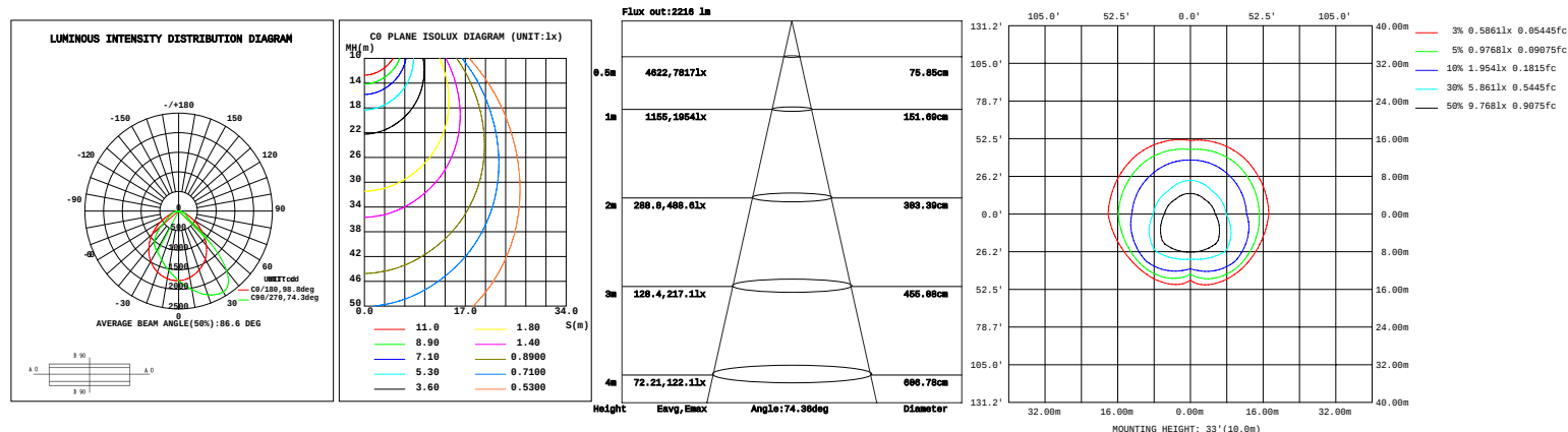
CIP-FWP2842567W27-345K (28W & 40000K)
