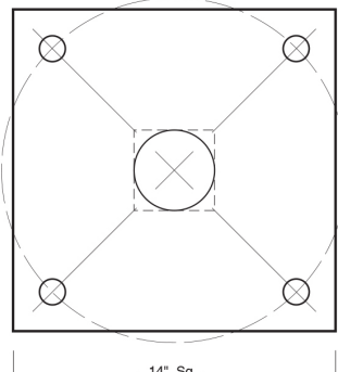
BF15 15" Bolt Circle
